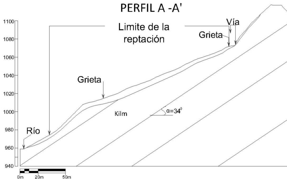
Figura 20. Esquema del movimiento, perfil desprendimiento
