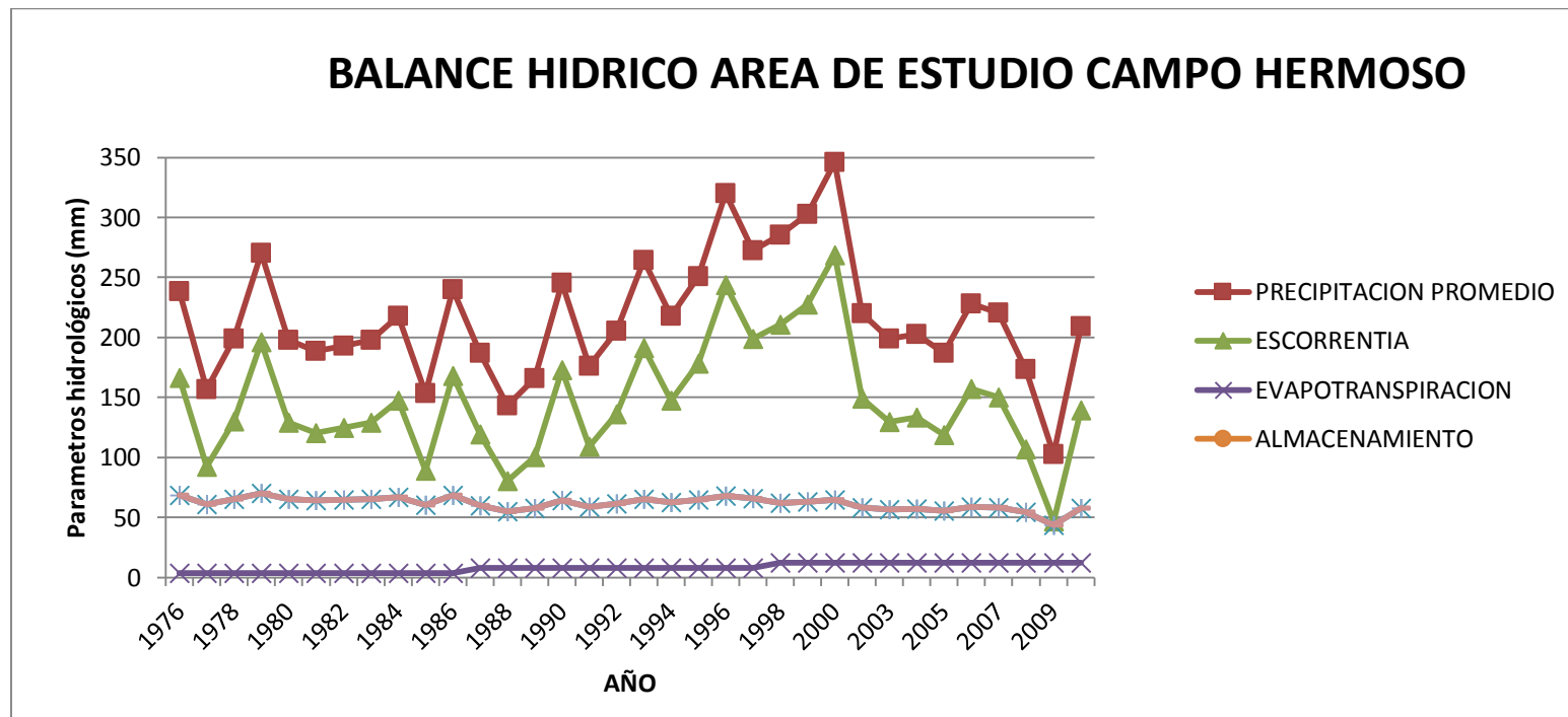
Figura 10. Comportamiento de las Curvas del Balance Hídrico.
