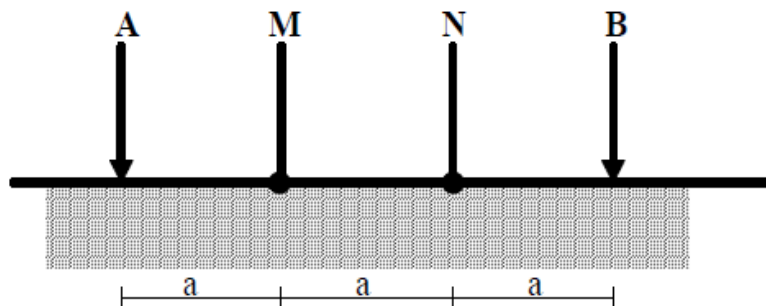
Figura 27. Dispositivo Wenner.
