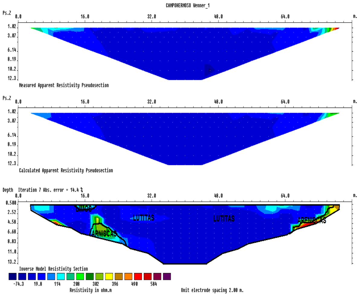
Figura 29. Perfil 1 tomografía.
