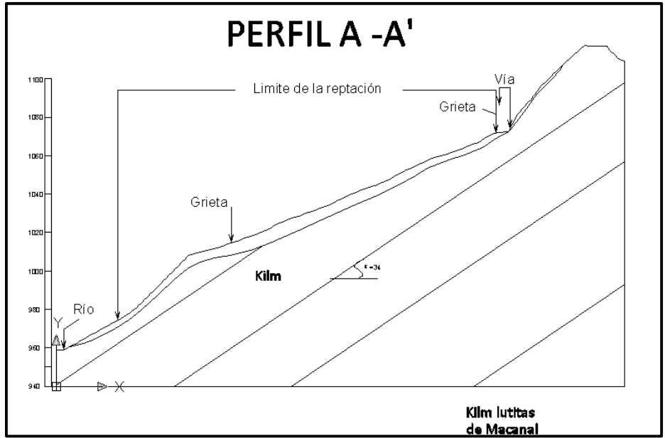
Figura 33. Perfil geológico AA'
