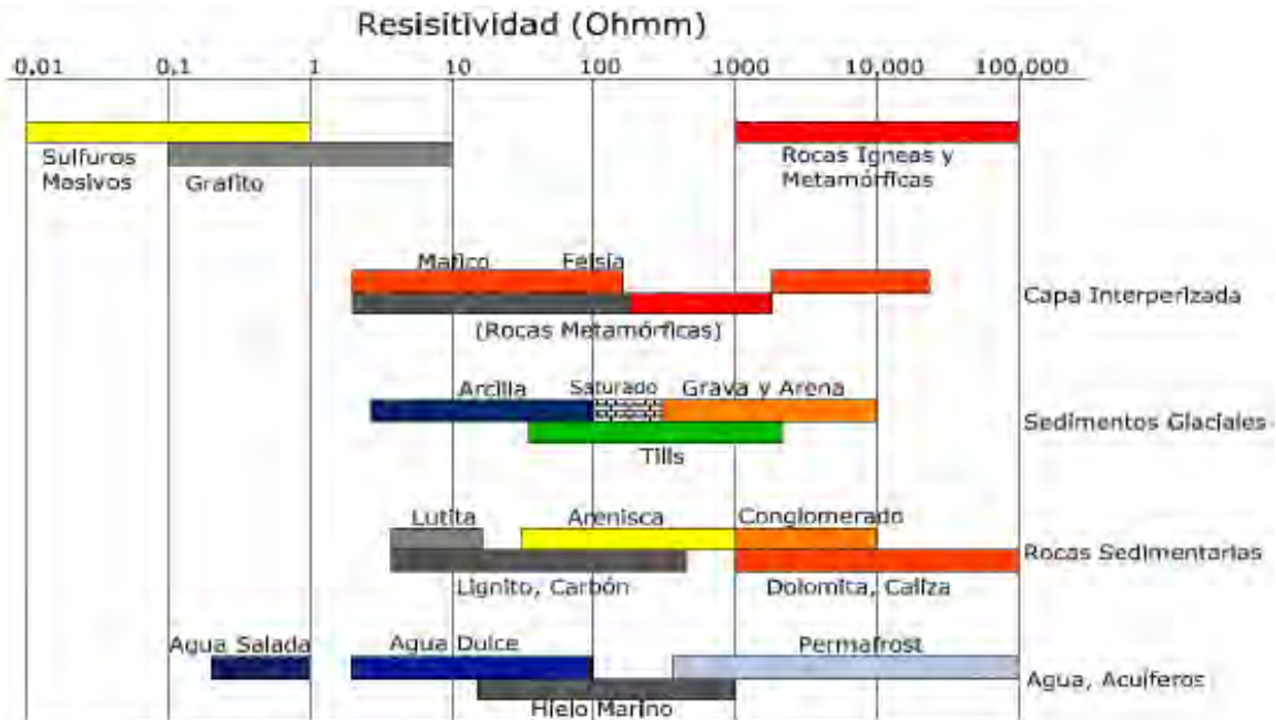
Figura 26. Rangos de resistividad para diferentes materiales.
