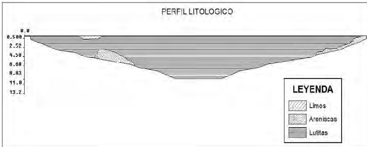
Figura 30. Perfil litológico 1
