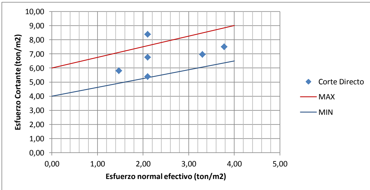
Figura 3. Análisis de los parámetros de resistencia (Sondeo 2)
