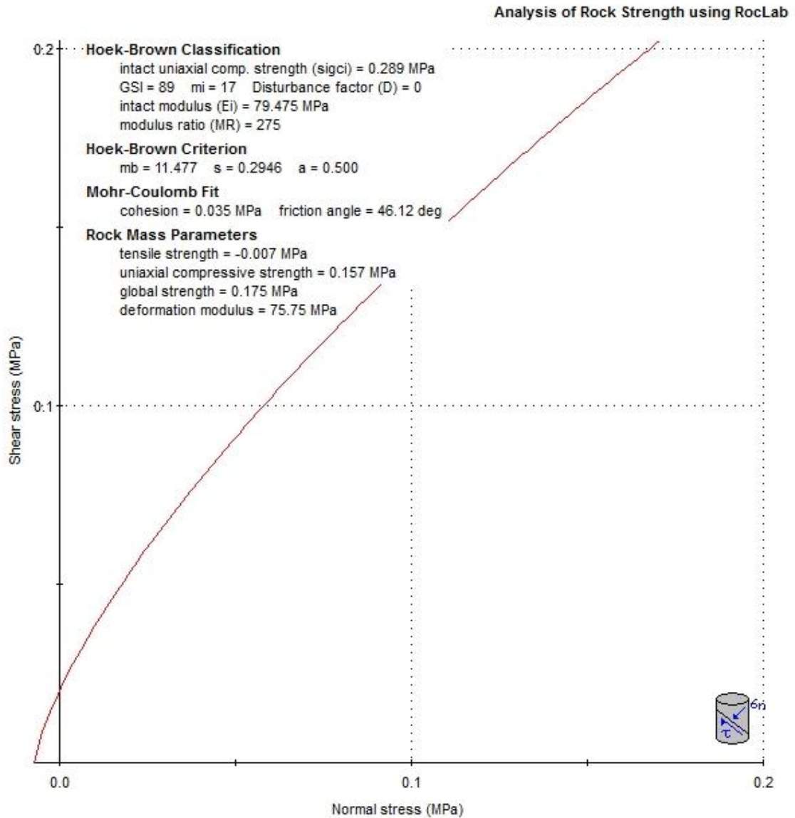
Figura 4. Salida gráfica del software RocLab 1.0 para la caracterización mecánica de la roca.
