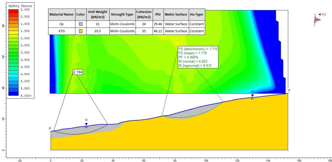
Figura 8. Distribución de los FS para el escenario actual en la condición extrema del Perfil 4.
