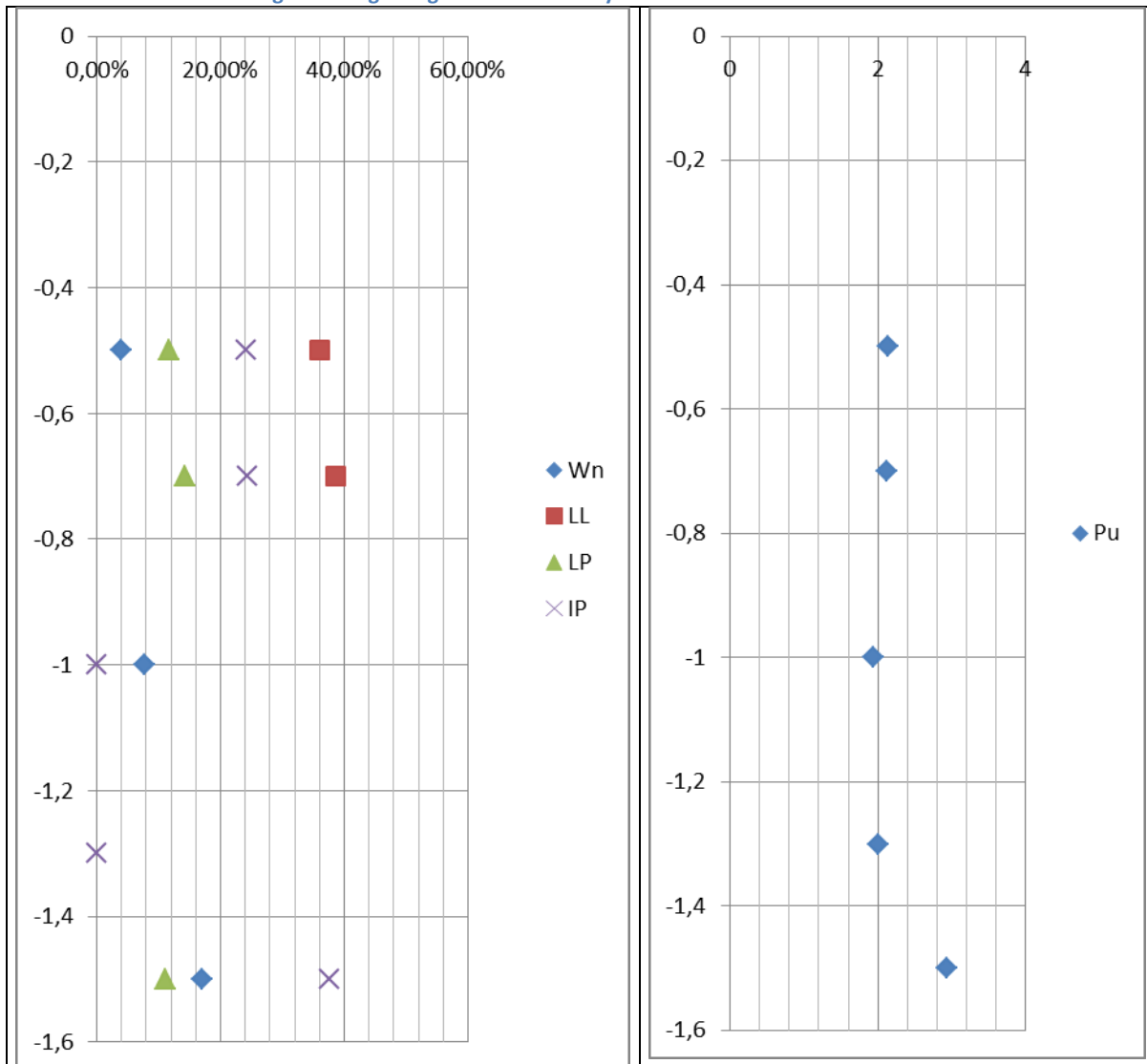
Figura 1. Registro gráfico de los ensayos de laboratorio del sondeo 2.
