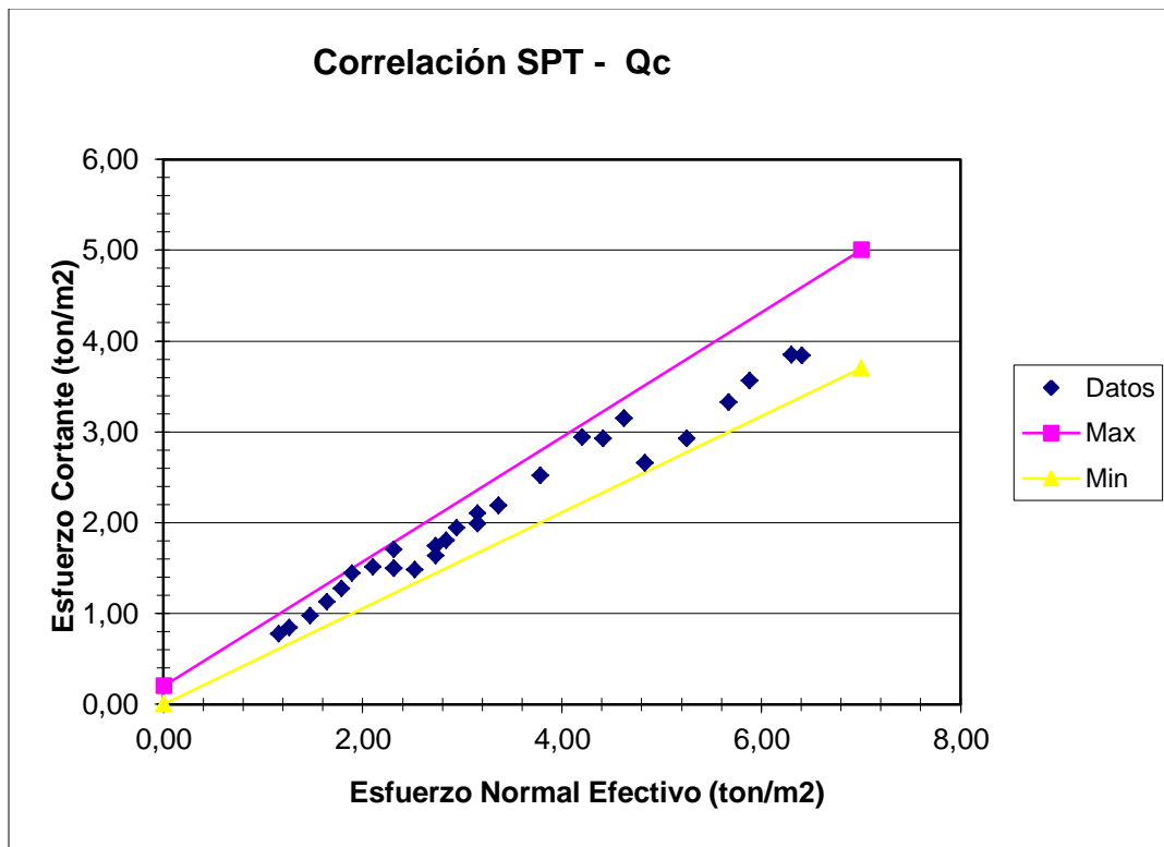
Figura 2. Análisis de los parámetros de resistencia a partir del SPT.
