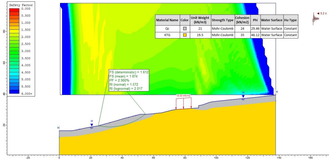
Figura 7. Distribución de los FS para el escenario actual en la condición extrema del Perfil 1.
