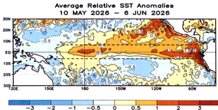
Figura 1 Anomalías de la temperatura relativa de la superficie del océano (SST, por sus siglas en inglés) en °C para el periodo comprendido entre el 10 de mayo y el 6 de junio de 2026. Fuente: NOAA.
